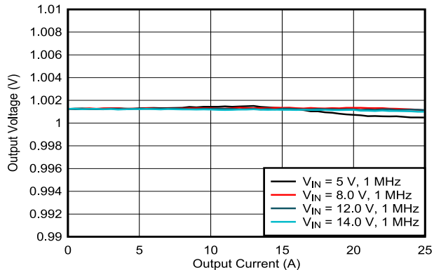
図 7-5. Load Regulation
