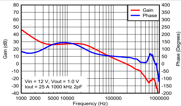
図 7-7. Bode Plot
