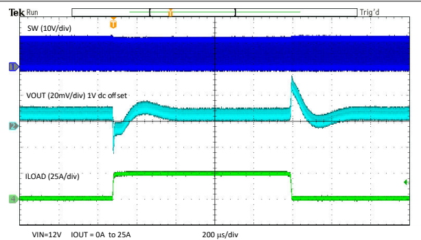
図 7-8. Load Transient
