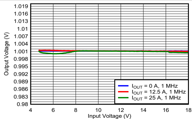
図 7-6. Line Regulation
