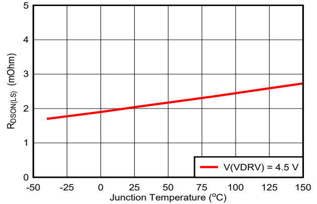
図 5-2. Low-Side FET R_{DS(on)}
