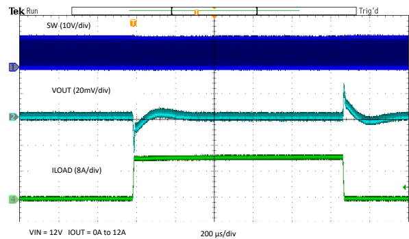
図 7-8. Load Transient
