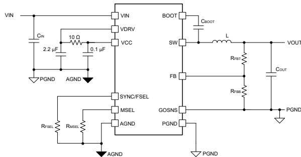
TPS543A22 のアプリケーション概略図
