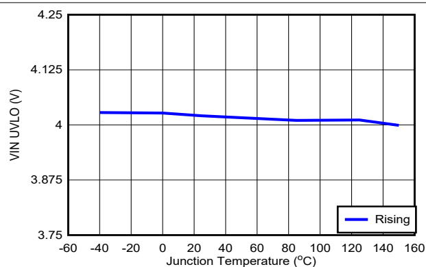
図 5-7. V_{IN} UVLO
