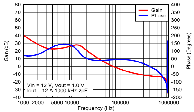
図 7-7. Bode Plot
