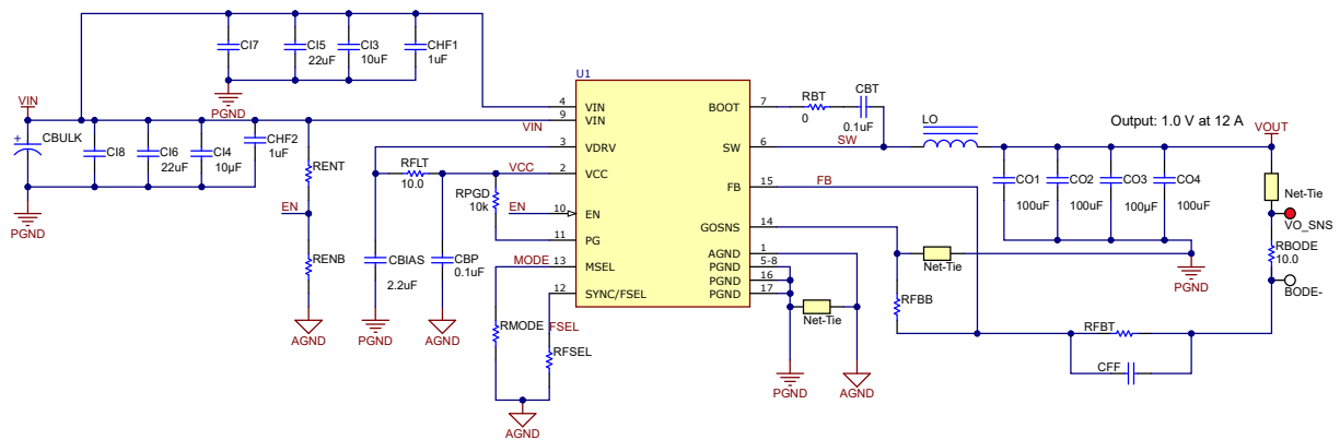
図 7-1. 12-V Input, 1.0-V Output, 1-MHz Schematic
