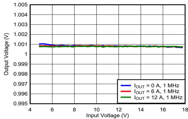
図 7-6. Line Regulation
