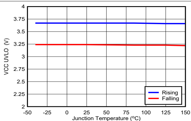
図 5-8. V_{CC} UVLO
