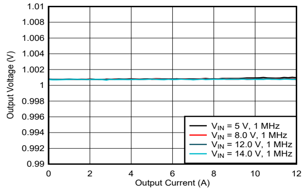
図 7-5. Load Regulation
