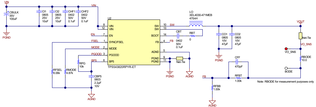
FIG 8-23. 12-V Input, 1.0-V Output, 1.5-MHz Schematic
