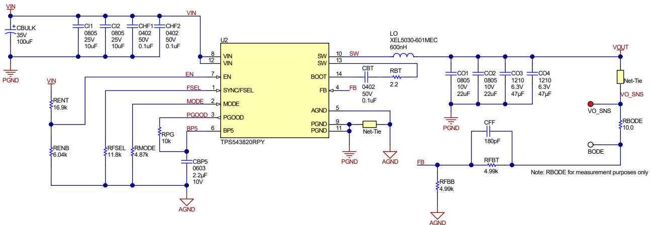
図 8-1. 12-V Input, 1.0-V Output, 1-MHz Schematic
