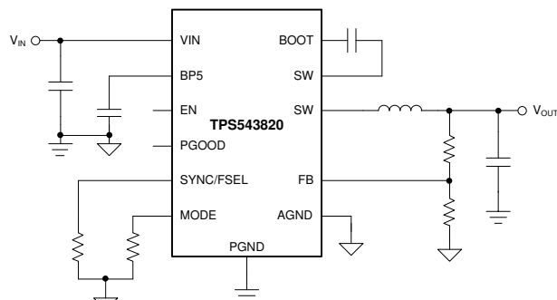
概略回路図
