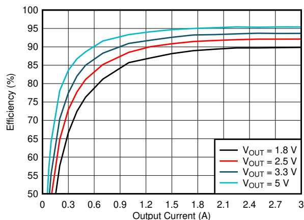
12 V in 、1MHz での効率
