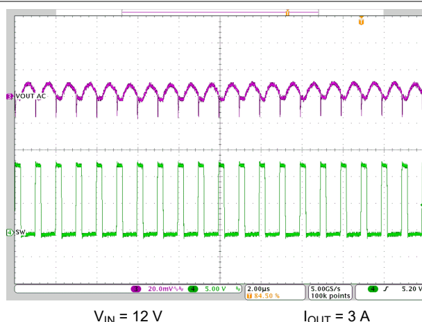
8-15. Output Ripple – 3-A Load
