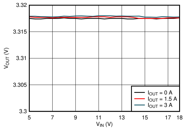
图 8-6. Line Regulation
