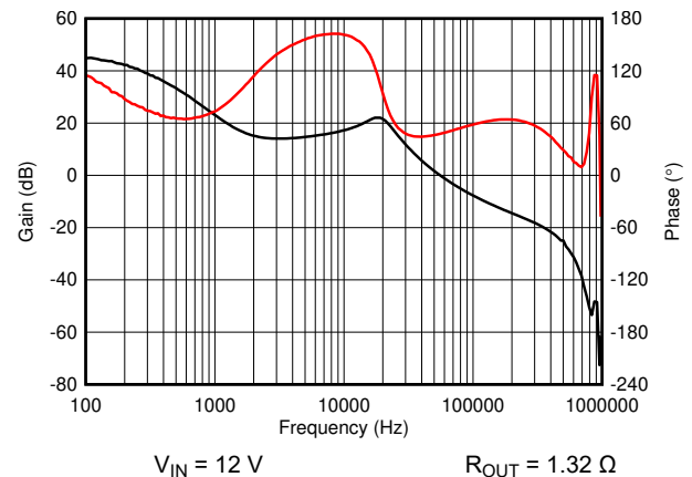
图 8-7. Bode Plot
