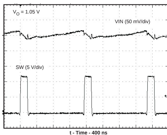
図 17. 入力電圧リップル ( I_O = 2A )
