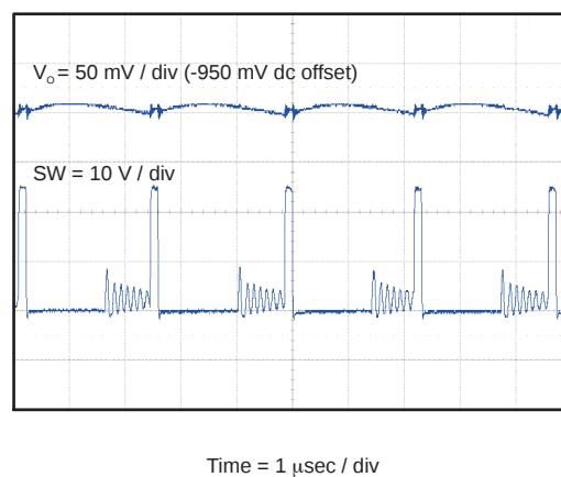
図 16. DCM出力電圧リップル ( I_O = 30mA )
