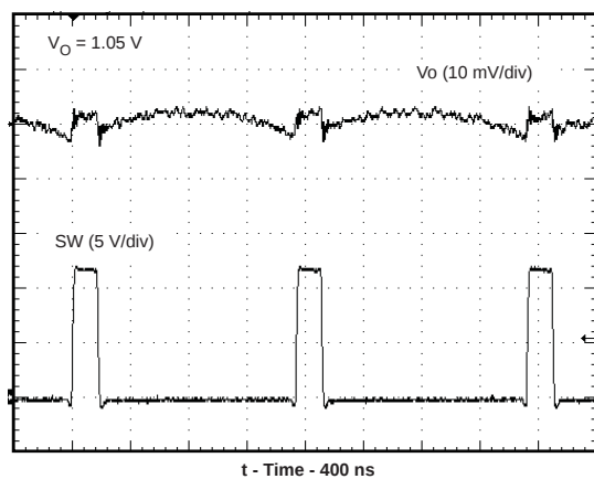
図 15. 出力電圧リップル ( I_O = 2A )
