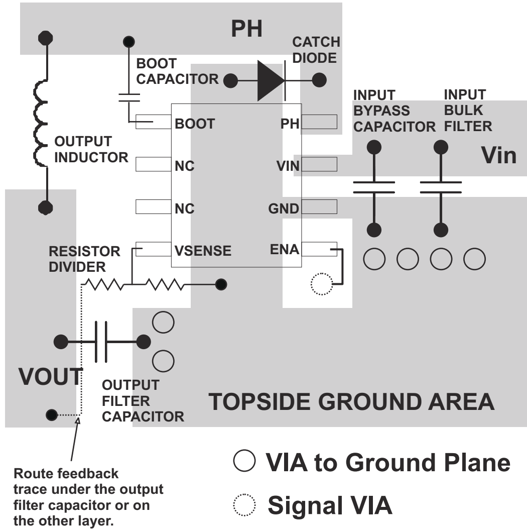
図 8-1. Design Layout
