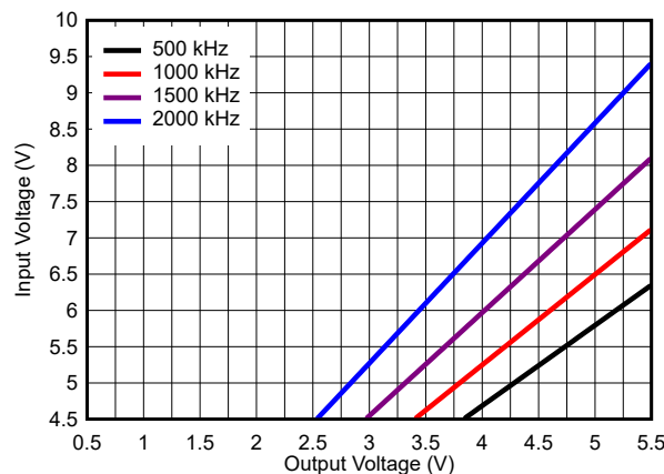
図 7-2. Minimum Input Voltage
