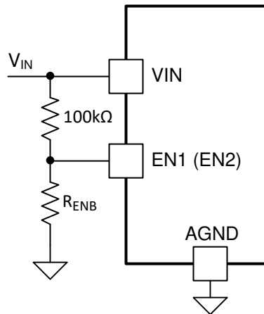
図 7-1. Enable ON/OFF Control
