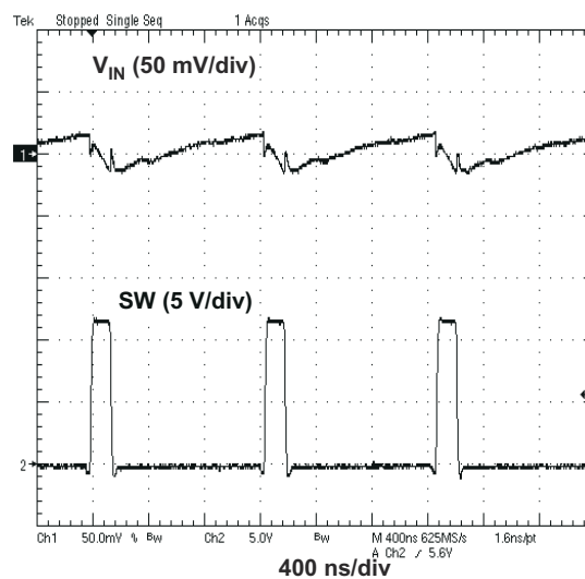
8-11. Input Voltage Ripple
