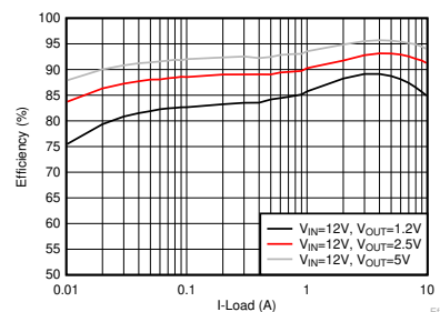
効率と出力電流との関係 (500kHz、ECO-mode)
