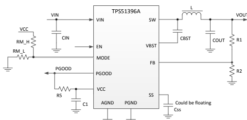
代表的なアプリケーション
