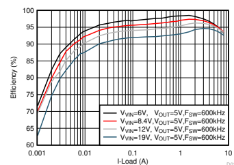
効率と出力電流との関係 (ECO-mode)
