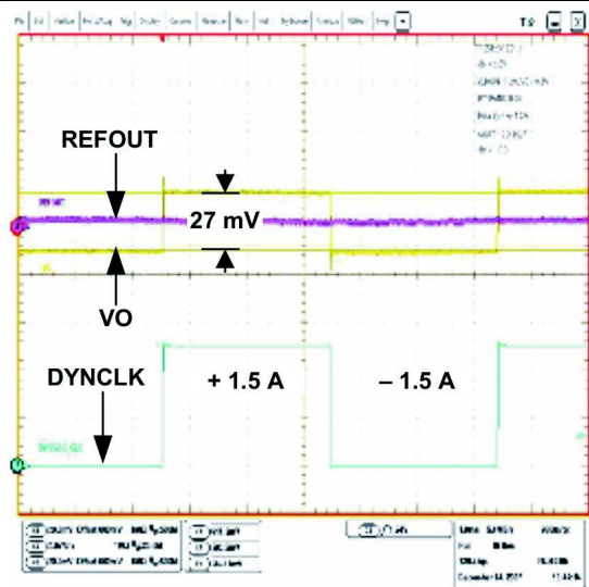
图 25. Transient Waveform
