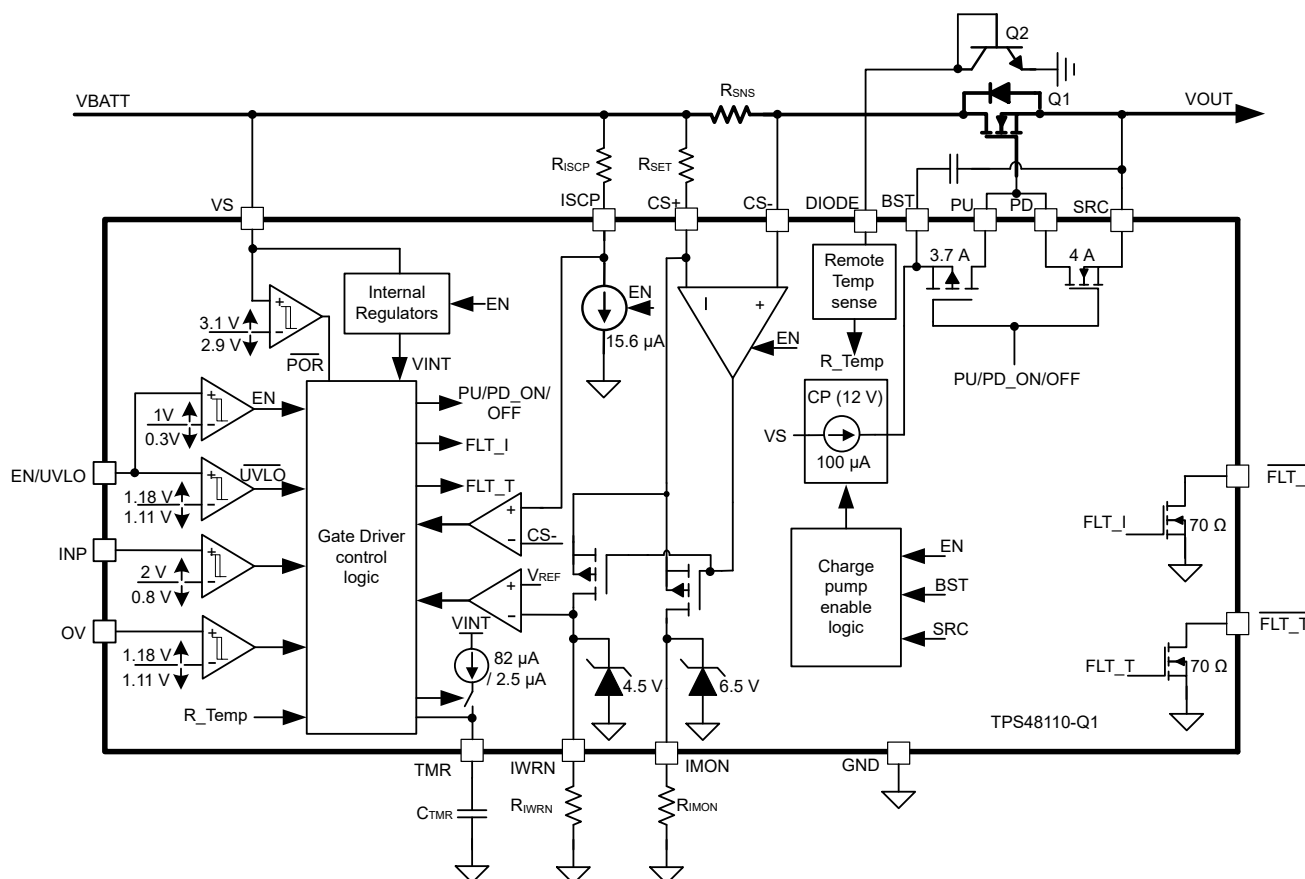
図 8-1. TPS48110-Q1 Functional Block Diagram
