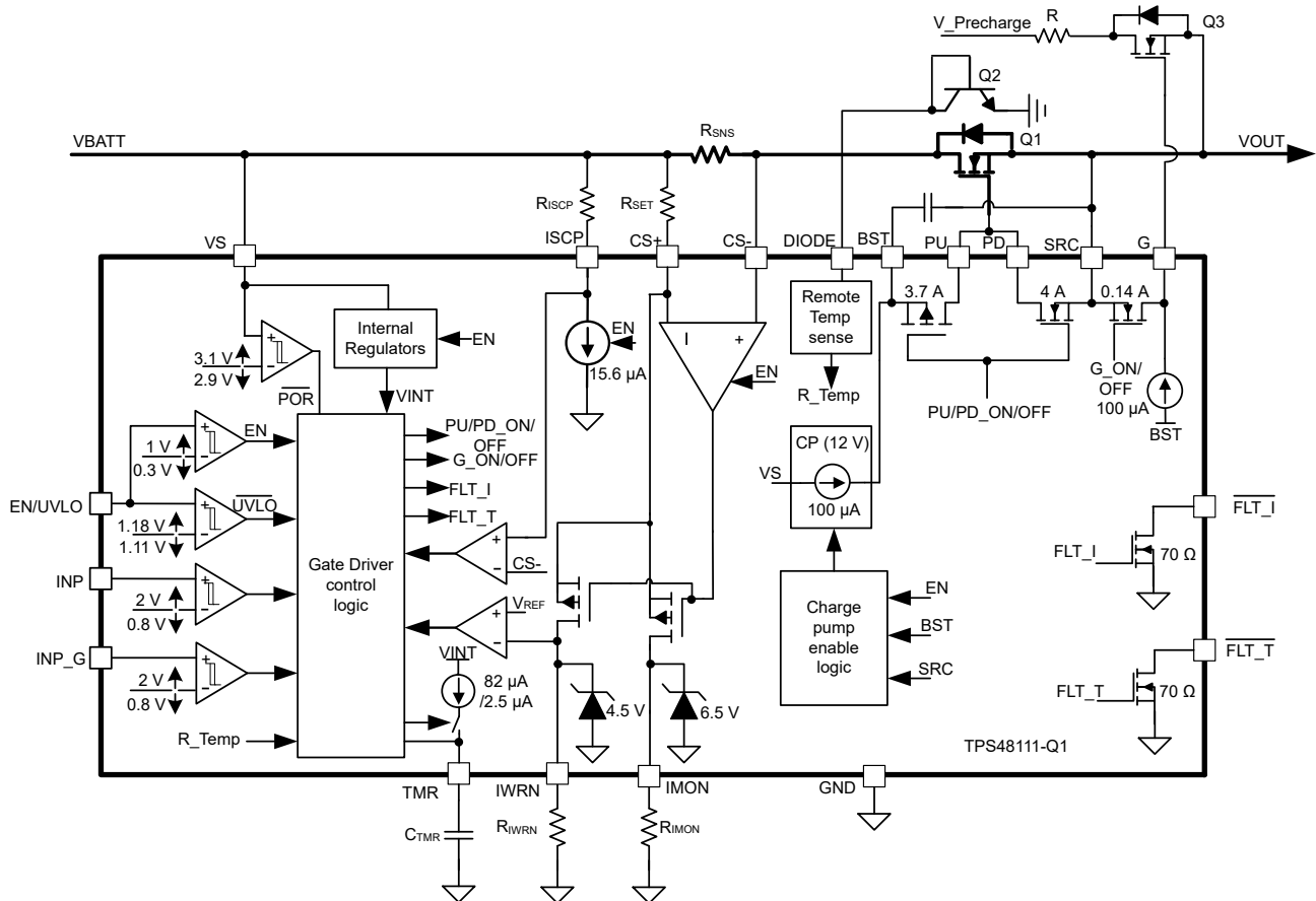
図 8-2. TPS4811-Q1 Functional Block Diagram
