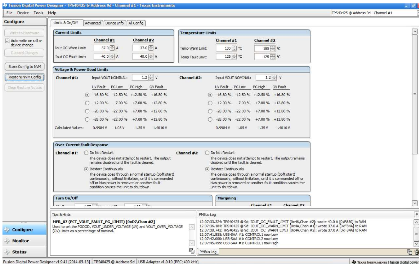
図 35. Fusion Digital Power Designerによるデバイス構成
