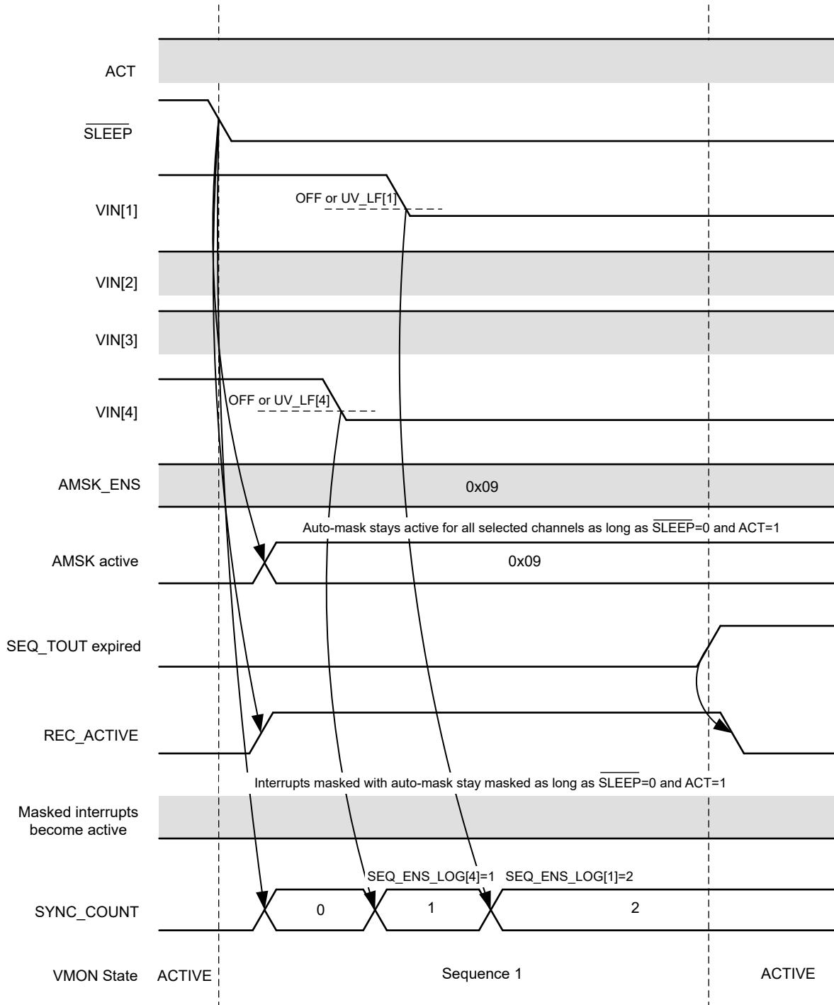
図 7-15. SLEEP 1→0 Transition
