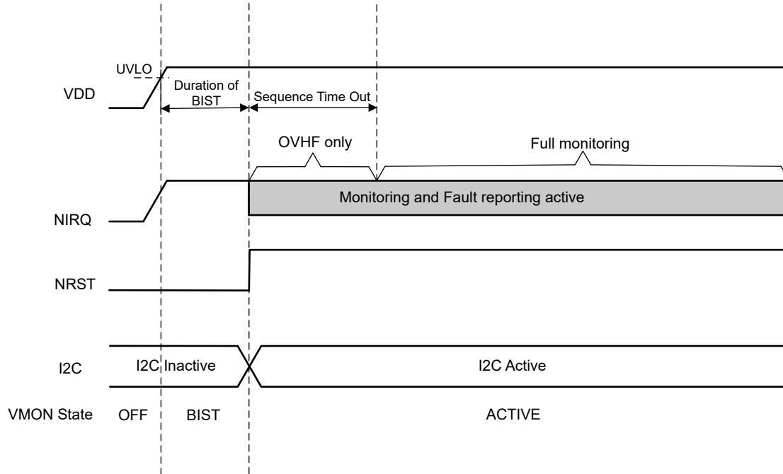
図 7-9. NRST スタートアップ時の動作
