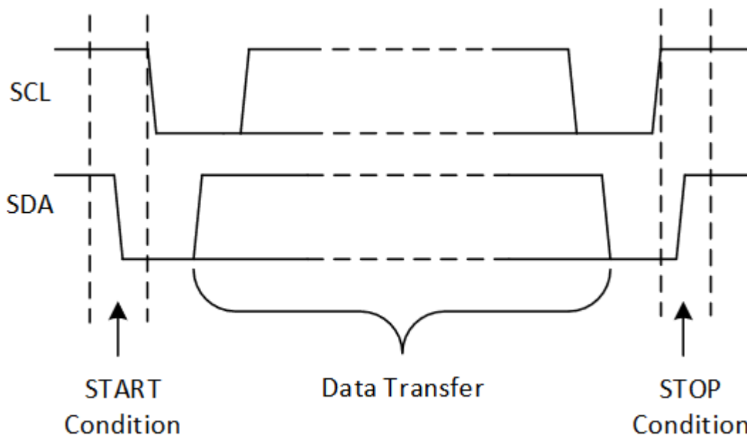
図 7-6. I 2 C の START 条件と STOP 条件
