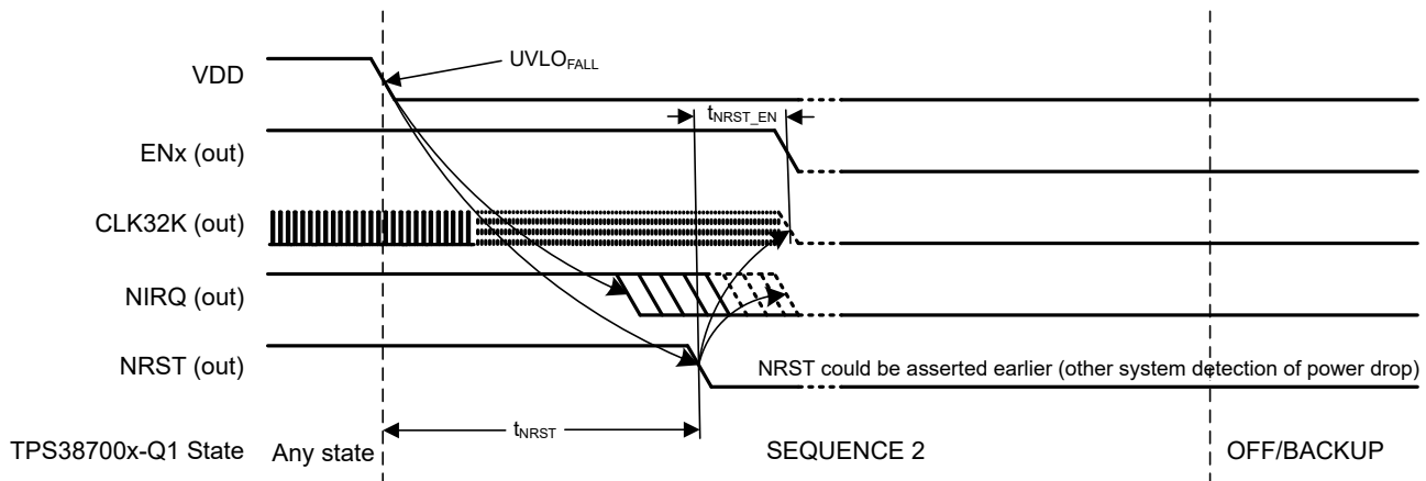
图 7-7. Emergency Power Down
