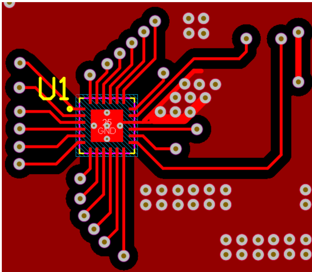
図 8-7. Recommended Layout
