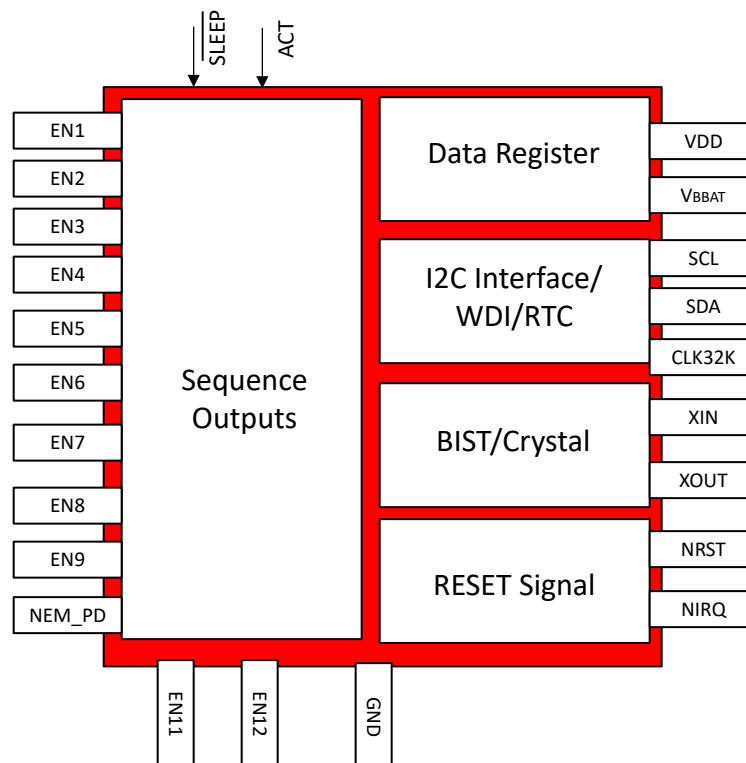
図 7-1. TPS38700-Q1 Block Diagram
