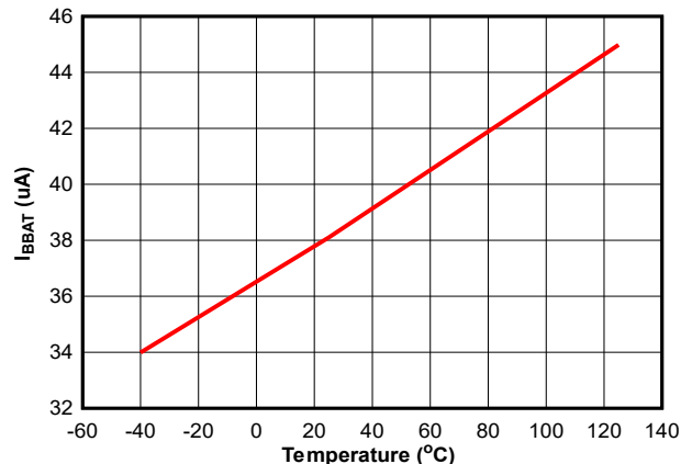
図 6-3. I_{BBAT} vs. Temperature
