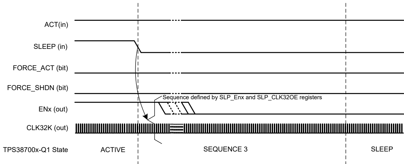
图 7-8. Sleep Entry
