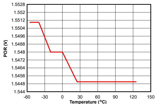
図 6-5. V_{POR} vs. Temperature
