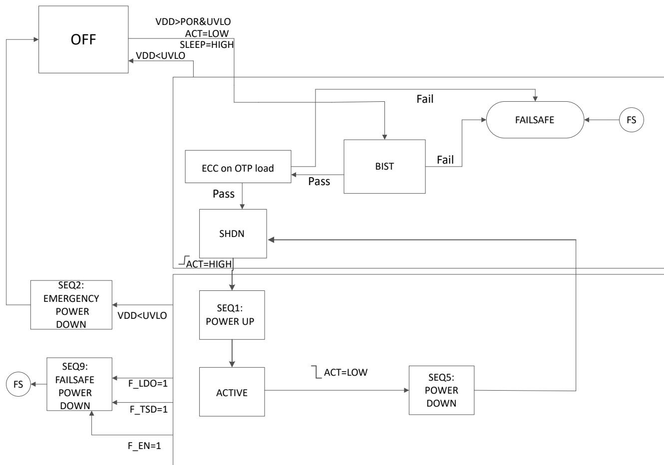
図 7-3. TPS38700-Q1 Simple Use Case
