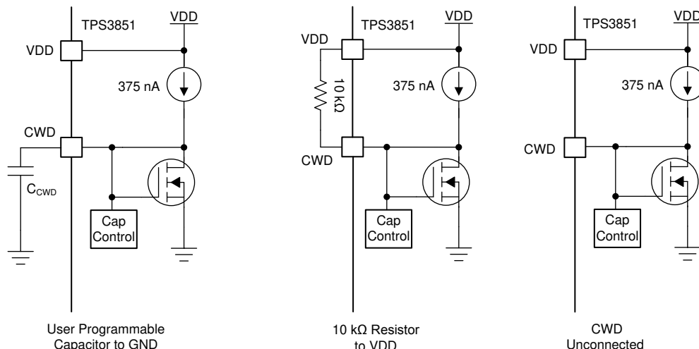
図 7-1. CWD 充電回路
