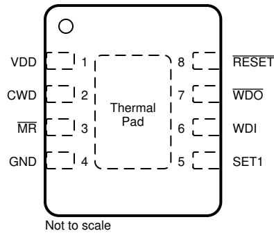
図 4-1. DRB パッケージ : TPS3851 3mm × 3mm VSON-8 上面図
