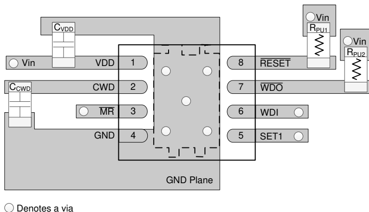
図 7-9. TPS3851 の推奨レイアウト
