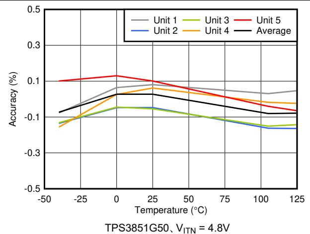
図 5-8. V_{ITN} + V_{HYST} の精度と温度との関係
