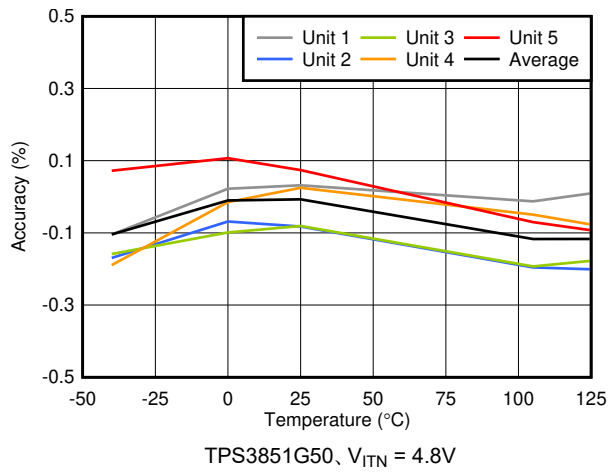
図 5-9. V_{ITN} 精度と温度との関係
