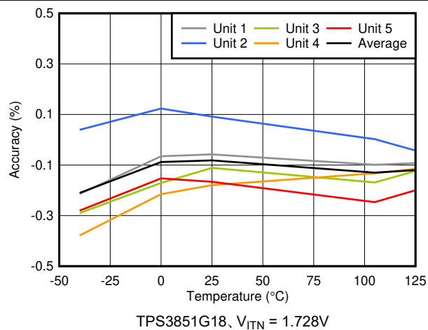
図 5-7. V_{ITN} 精度と温度との関係
