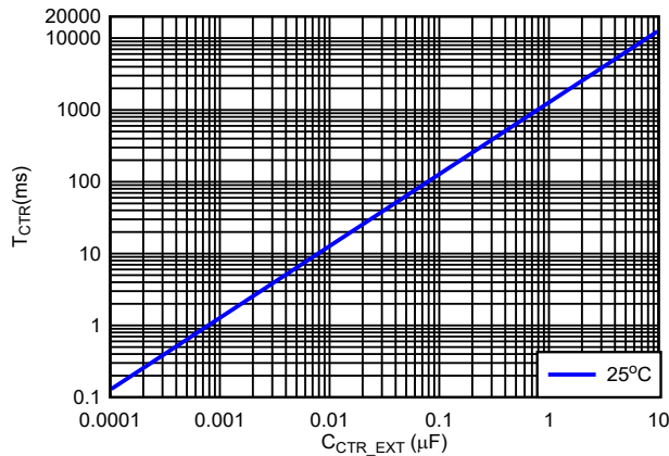
図 7-4. T_{CTR} vs C_{CTR}
