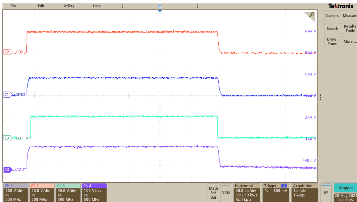
図 8-2. TPS37100 waveform
