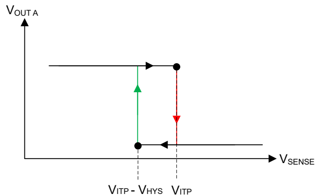
図 7-4. Hysteresis (Overvoltage Active-Low)
