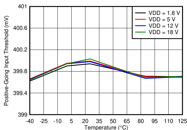
立ち上がり入カスレッシュホールド電圧 ( V_{IT+} ) と温度との関係
