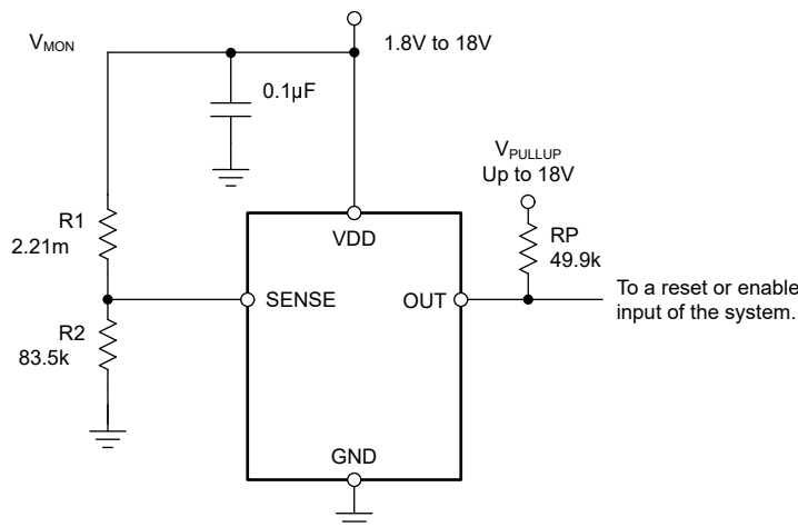
図 7-4. Wide VIN Voltage Monitor
