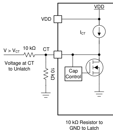
図 9-3. RESET Latch Circuit
