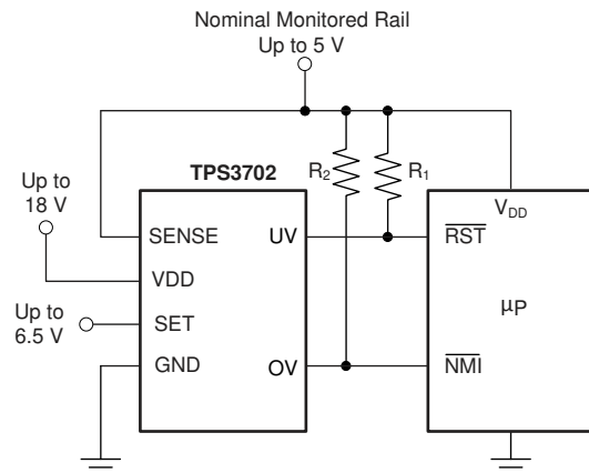
代表的なアプリケーション回路
