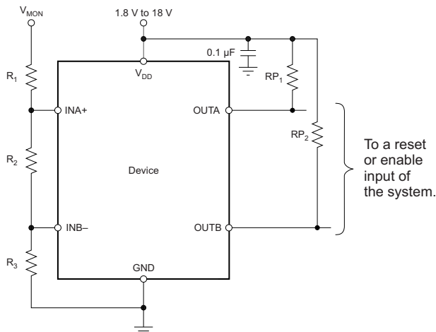
概略回路図
