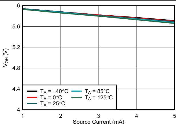
7-16. RESET V_{OH} vs I_{source} , V_{DD} = 6.0\text{ V}
