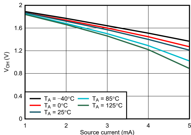
7-15. WDO V_{OH} vs I_{source} , V_{DD} = 2.0\text{ V}
