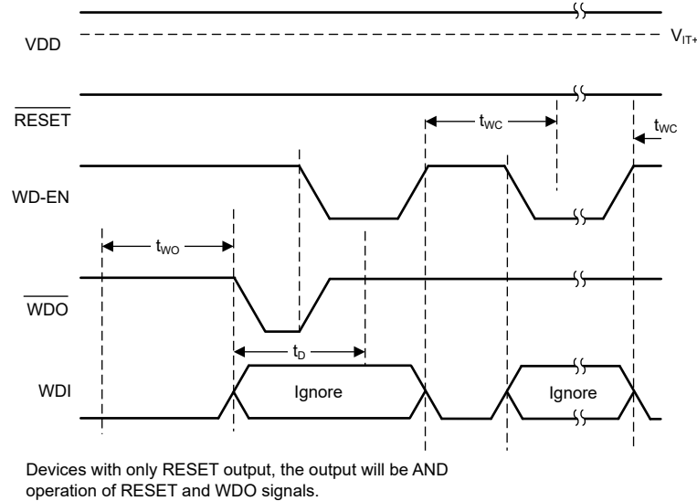
図 8-7. Watchdog Enable: WD-EN Pin Control
