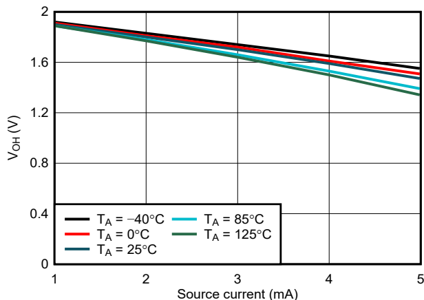
7-14. RESET V_{OH} vs I_{source} , V_{DD} = 2.0\text{ V}
