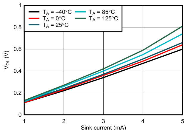
図 6-10. RESET V_{OL} と I_{sink} との関係、 V_{DD} = 1.5\text{V}
