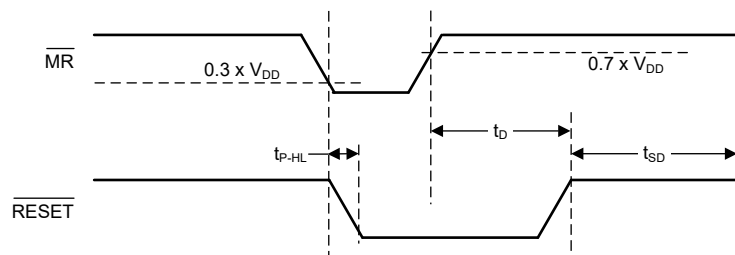
図 7-14. \overline{\text{MR}} ピンの応答
