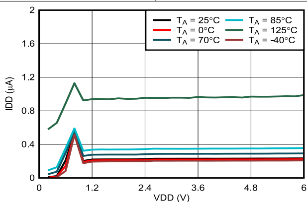
図 6-18. 電源電流と電源電圧との関係
