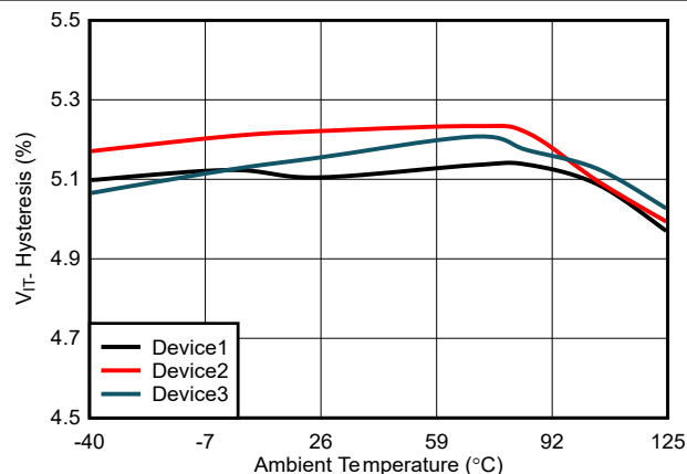
図 6-4. V_{IT} のヒステリシスと温度との関係
