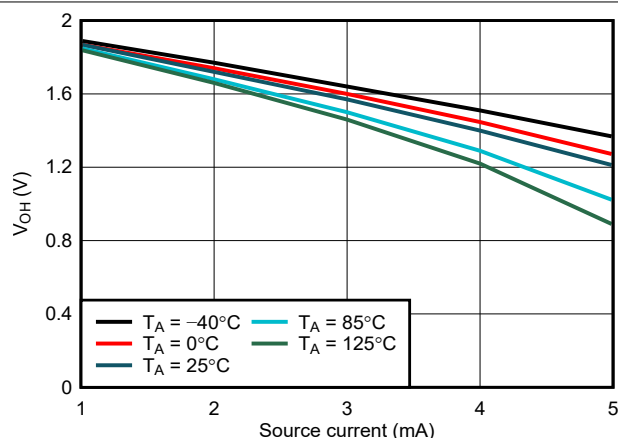
図 6-15. WDO V_{OH} と I_{source} との関係、 V_{DD} = 2.0\text{V}
