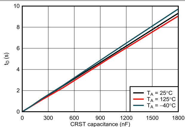
図 6-9. t_D と容量との関係
