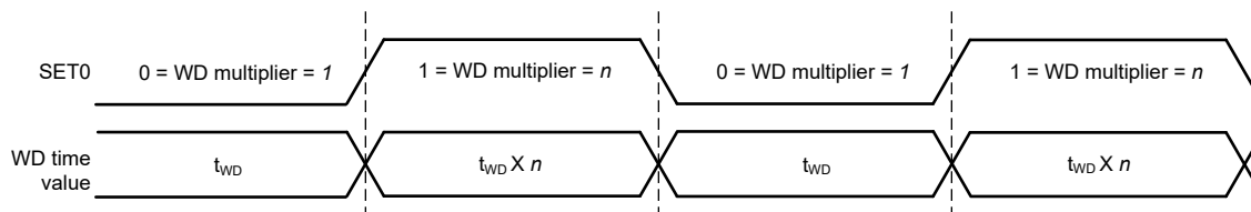
図 7-12. 2 本の SET ピンによるウォッチドッグ動作
