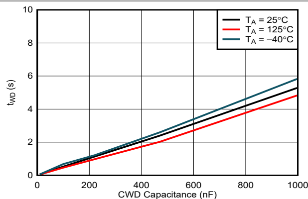
図 6-8. t_{WD} と容量との関係
