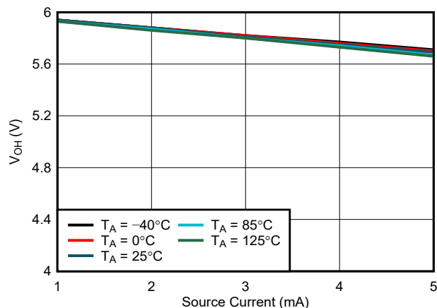
図 6-16. RESET V_{OH} と I_{source} との関係、 V_{DD} = 6.0\text{V}
