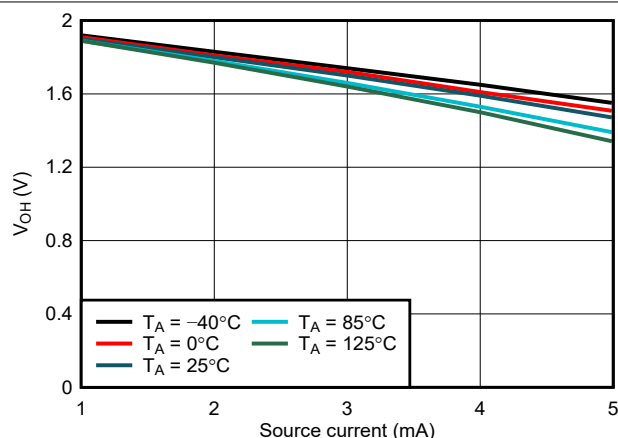
図 6-14. RESET V_{OH} と I_{source} との関係、 V_{DD} = 2.0\text{V}
