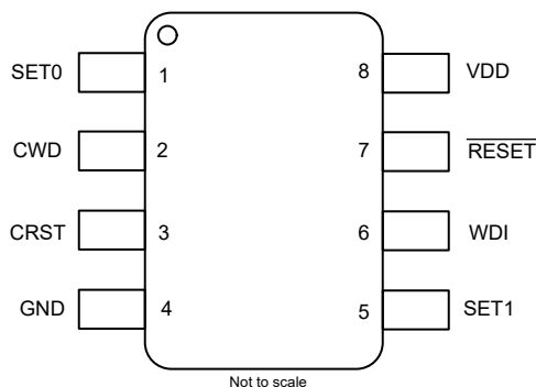
図 5-2. ピン構成オプション B DDF パッケージ、8 ピン SOT-23、 TPS35 上面図
