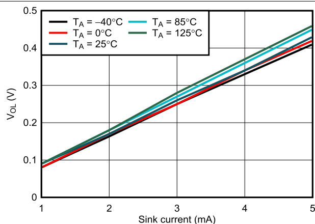
図 6-12. RESET V_{OL} と I_{sink} との関係、 V_{DD} = 3.3\text{V}
