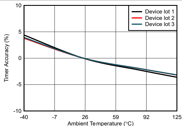
図 6-6. タイマの精度と温度との関係
