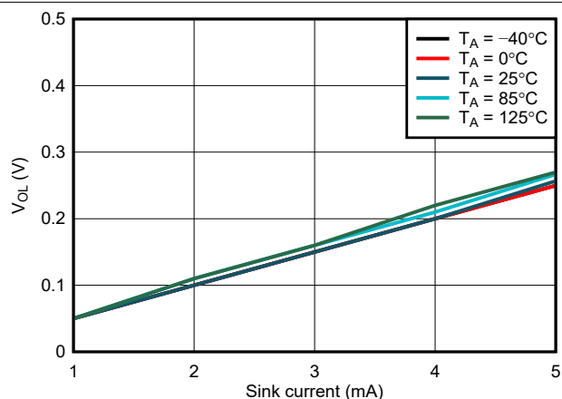
図 6-13. WDO V_{OL} と I_{sink} との関係、 V_{DD} = 3.3\text{V}
