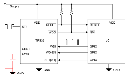
代表的なアプリケーション回路
