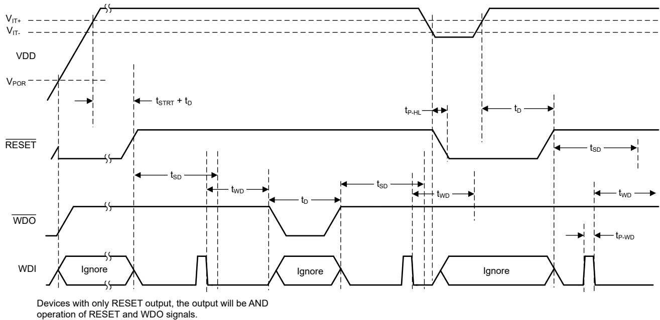
図 7-7. 電圧スーバイザのタイミング図
