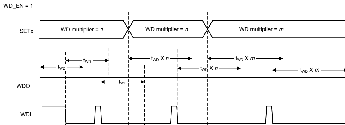
図 7-11. SETx ピンのステータスによるウォッチドッグ動作
