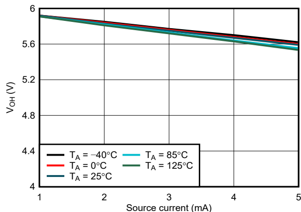
図 6-17. WDO V_{OH} と I_{source} との関係、 V_{DD} = 6.0\text{V}
