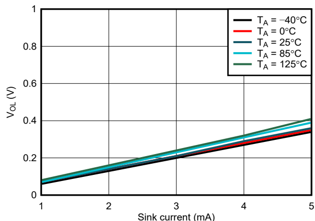
図 6-11. WDO V_{OL} と I_{sink} との関係、 V_{DD} = 1.5\text{V}
