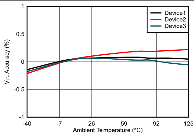
図 6-2. V_{IT} の精度と温度との関係
