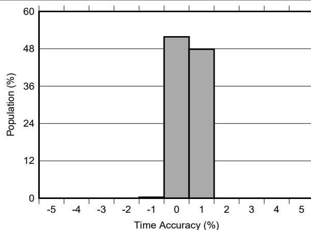
図 6-7. タイマの精度ヒストグラム
