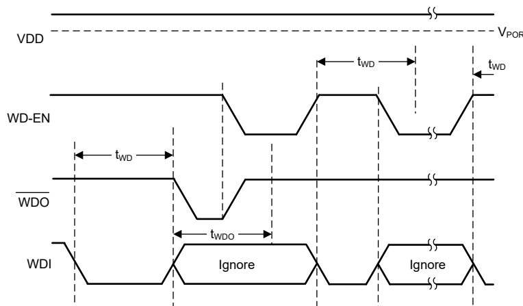
図 7-5. ウォッチドッグのイネーブル : WD-EN ピンの制御
