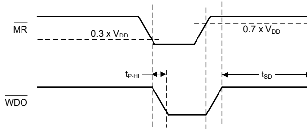
図 7-10. \overline{\text{MR}} ピンの応答
