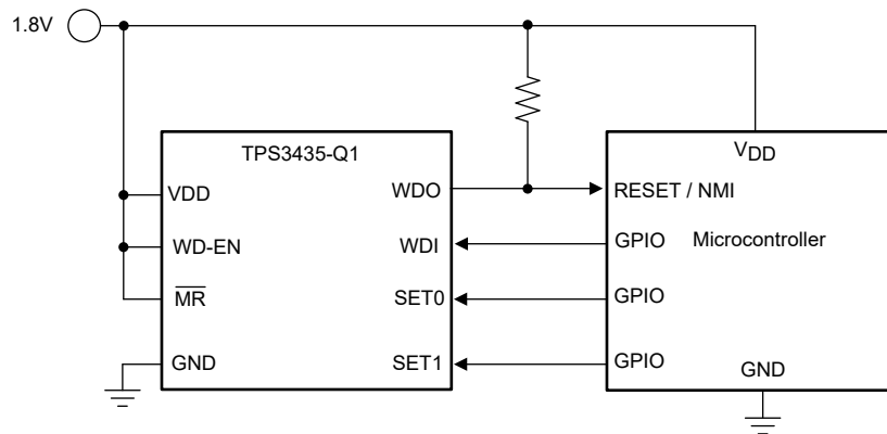
図 8-1. マイクロコントローラ ウォッチドッグ監視回路
