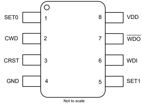
図 5-2. ピン構成オプション B DDF パッケージ、8 ピン SOT-23、 TPS3435-Q1 上面図
