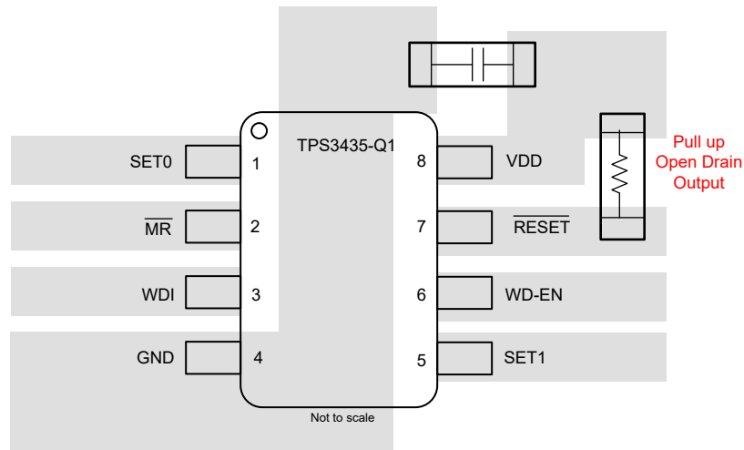
図 8-3. 以下のデバイスのピン配置 C の代表的なレイアウト： TPS3435-Q1
