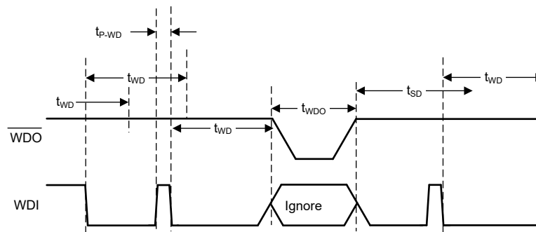
図 7-4. タイムアウトウォッチドッグタイマの動作
