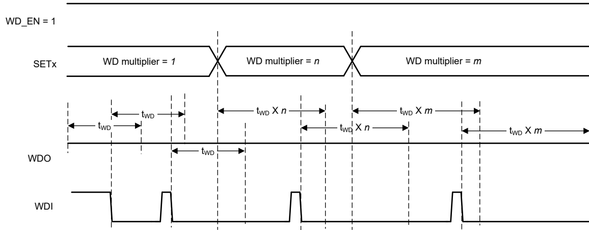
図 7-7. SETx ピンのステータスによるウォッチドッグ動作
