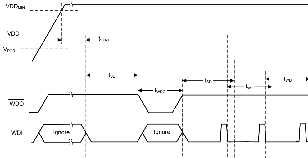
図 7-6. t_{SD} フレームの動作
