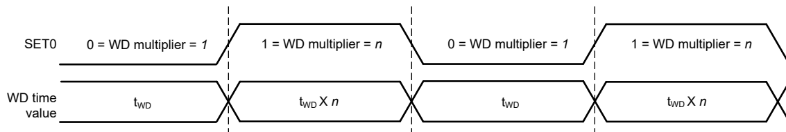
図 7-8. 2 本の SET ピンによるウォッチドッグ動作
