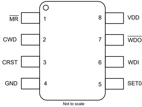
図 5-1. ピン構成オプション A DDF パッケージ、8 ピン SOT-23、 TPS3435-Q1 上面図
