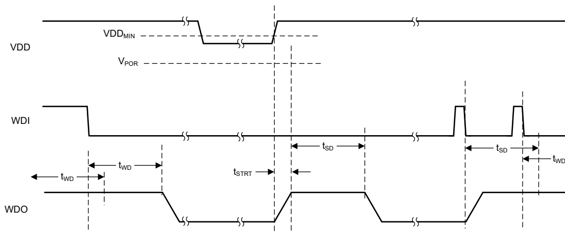
図 7-11. 出力ラッチのタイミング動作
