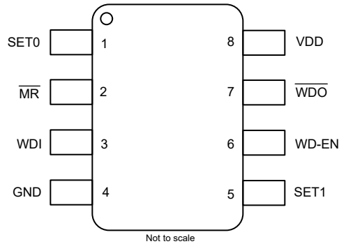
図 5-3. ピン構成オプション C DDF パッケージ、8 ピン SOT-23、 TPS3435-Q1 上面図
