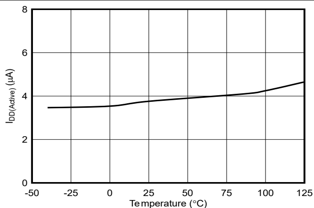
図 6-6. アクティブ電流と温度との関係 (アクティブ Low のプッシュボタン入力)
