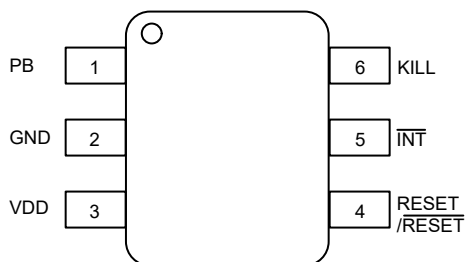
図 5-4. ピン構成オプション TPS3424 DRL パッケージ 、6 ピン SOT-5X3 上面図
