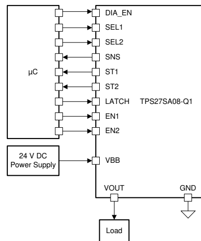
簡略回路図
