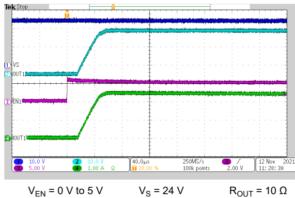
图 7-9. Turn-on Time ( T_{ON} )
