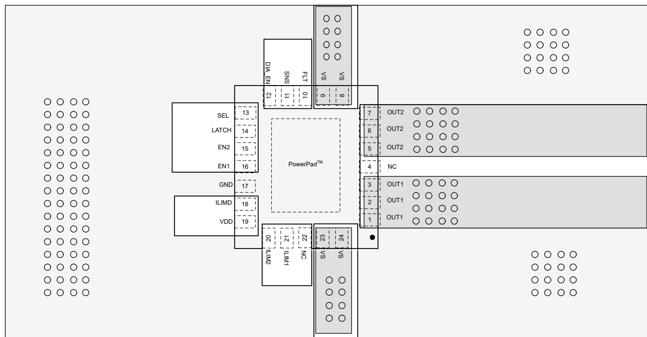
✎ 10-10. Layout Example
