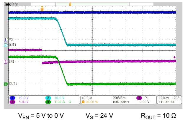
图 7-10. Turn-off Time ( T_{OFF} )
