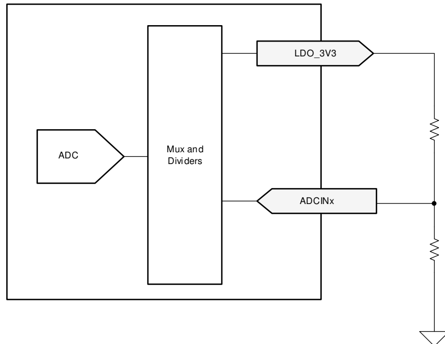
図 7-13. ADCINx Resistor Divider
