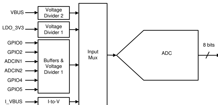
図 7-14. SAR ADC
