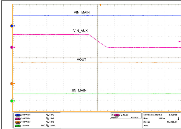
図 9-15. VIN_AUX Brownout Condition
