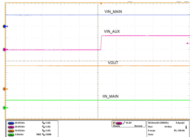
図 9-16. VIN_AUX Power Recovery
