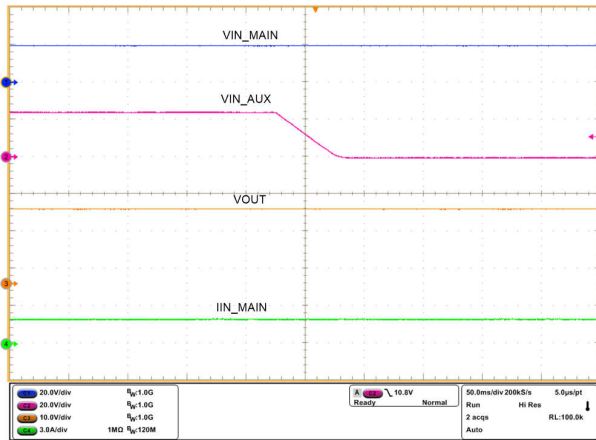
図 9-15. VIN_AUX Brownout Condition
