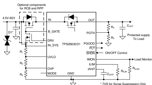
概略回路図
