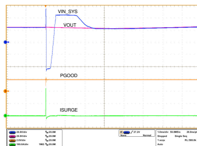
24V 電源での IEC61000-4-5 サージ性能
