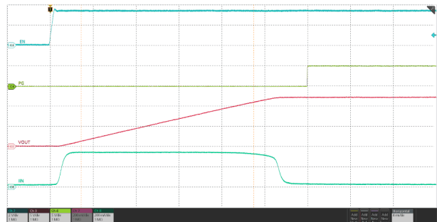
図 6-32. Input Hot-Plug
