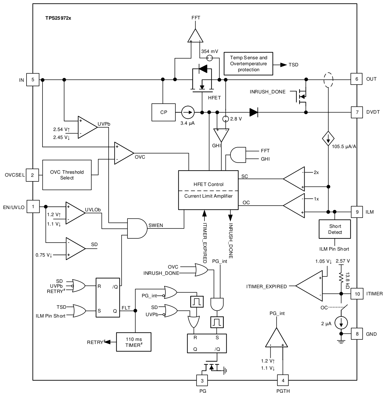
図 7-2. TPS25972x Block Diagram
