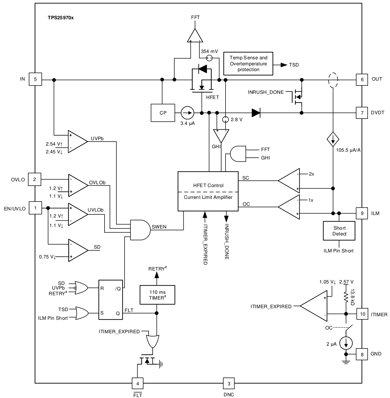
図 7-1. TPS25970x Block Diagram
