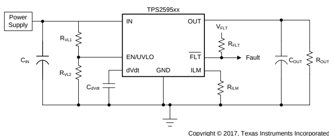
概略回路図
