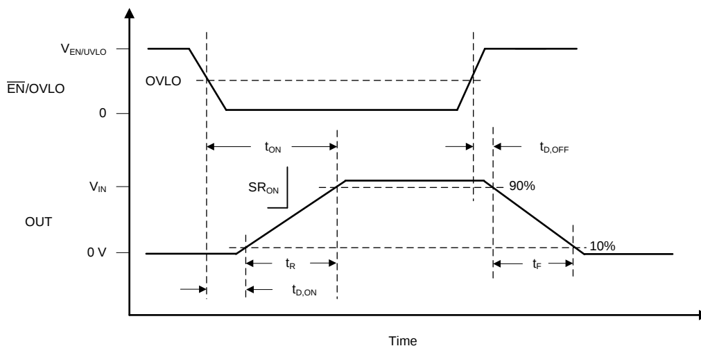
图 2. TPS2595x3 Switching Times
