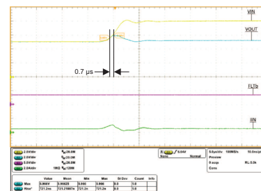
TPS25953x過電圧クランプの応答時間
