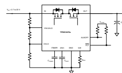
概略回路図
