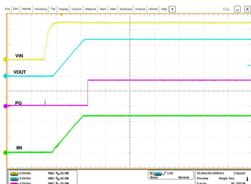
图 7-40. Input Hot-Plug
