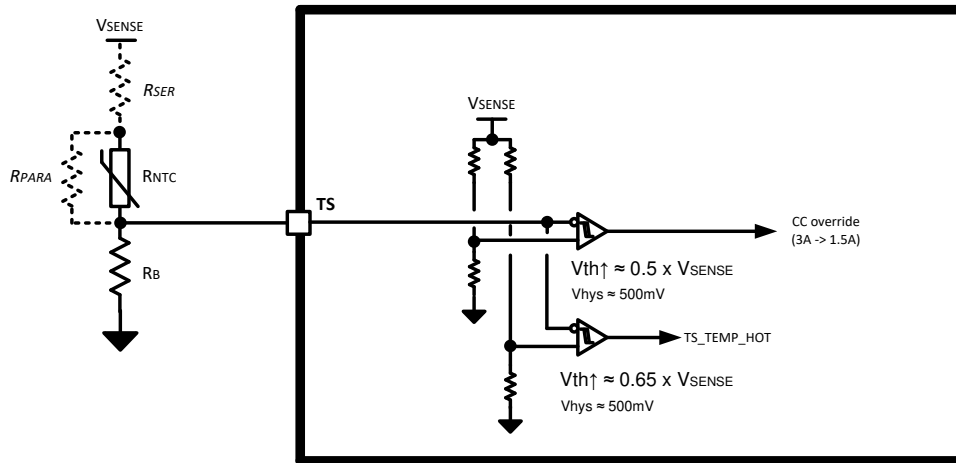
FIG 10-16. TS Input
