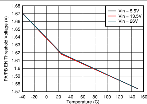
FIG 8-4. Precision USB PA/PB Enable Threshold
