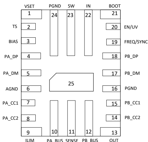
7-1. TPS25850-Q1 RPQ Package 25-Pin (QFN) Top View
