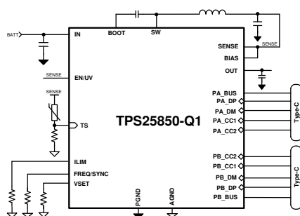
TPS25850-Q1 の概略回路図
