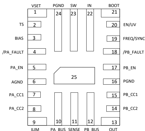
7-3. TPS25852-Q1 RPQ Package 25-Pin (QFN) Top View
