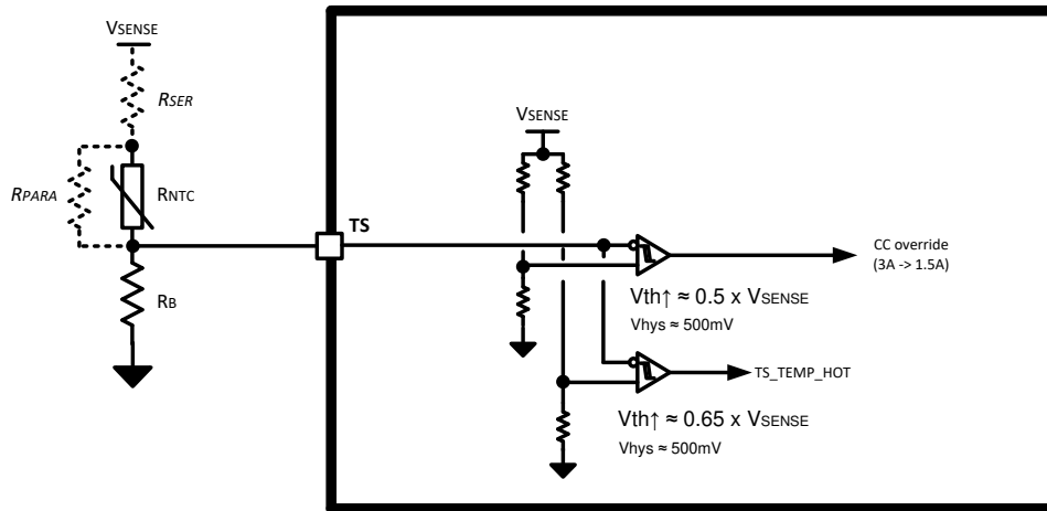
FIG 10-16. TS Input
