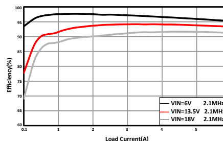
効率と出力電流との関係
