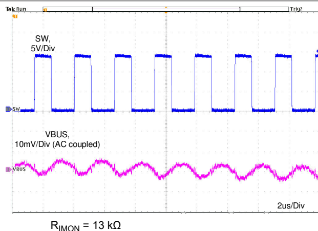
11-13. 3.5-A Output Ripple
