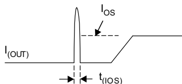
FIG 9-3. Short-Circuit Parameters
