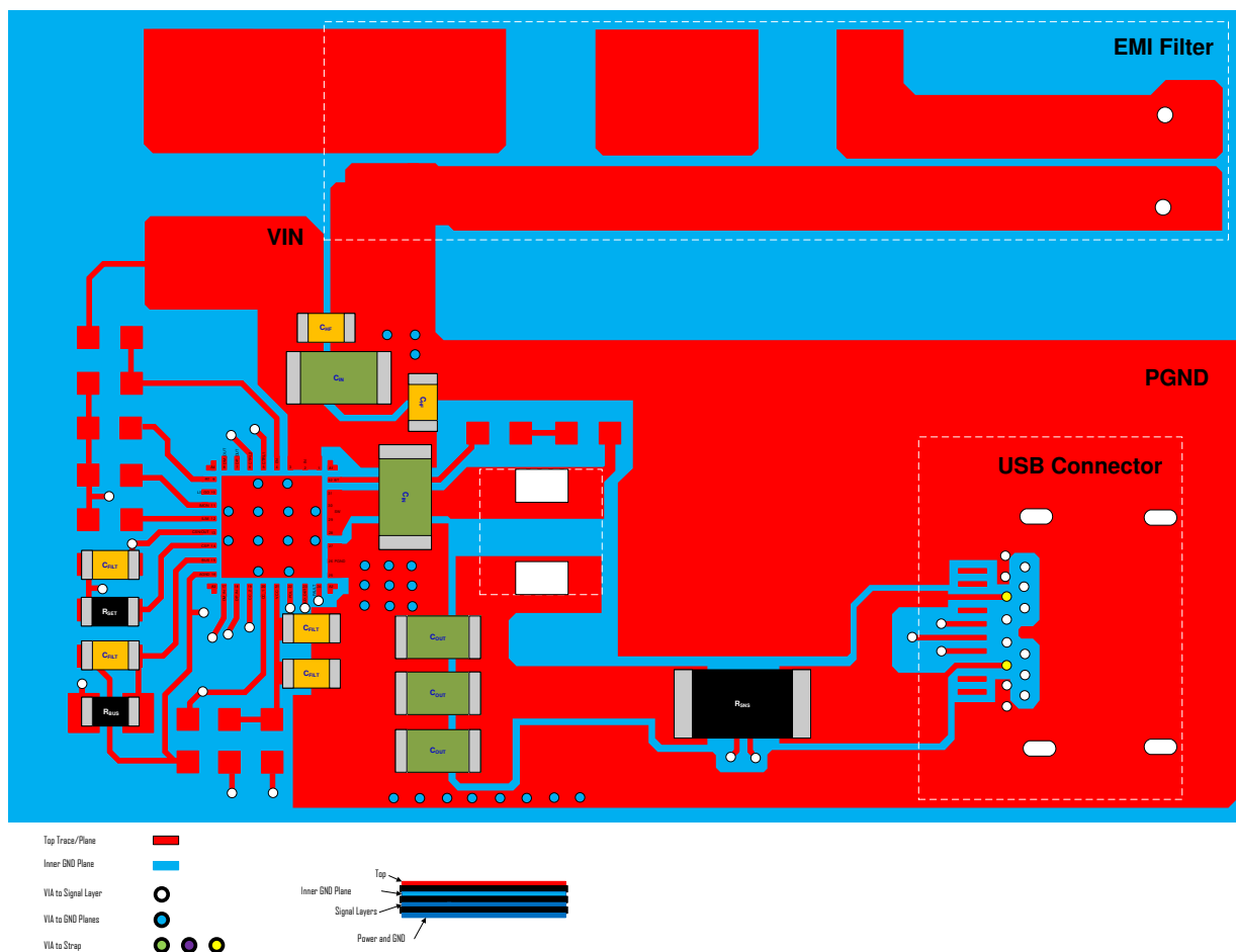
图 13-1. Layout
