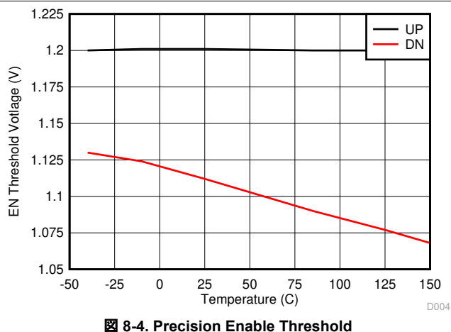
8-4. Precision Enable Threshold
