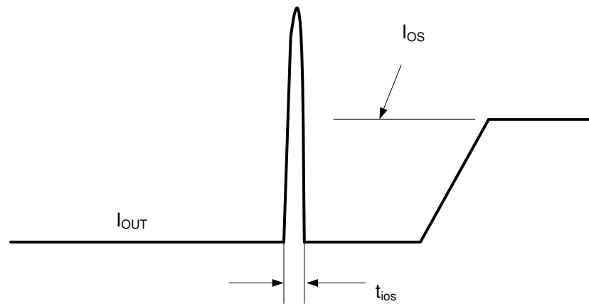
図 1. Output Short Circuit Parameter Diagram
