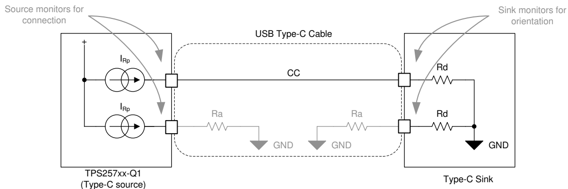
図 8-29. Type-C Cable
