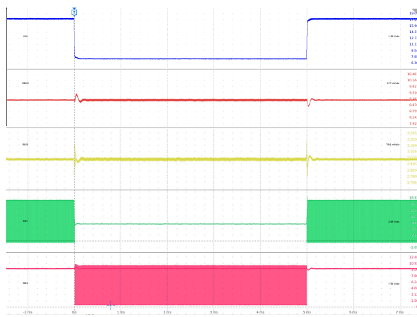
図 9-35. Line Transient: V_{BUS} = 20\text{ V}
