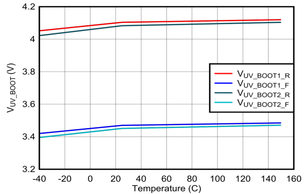
図 6-22. BOOTx UVLO vs Temperature
