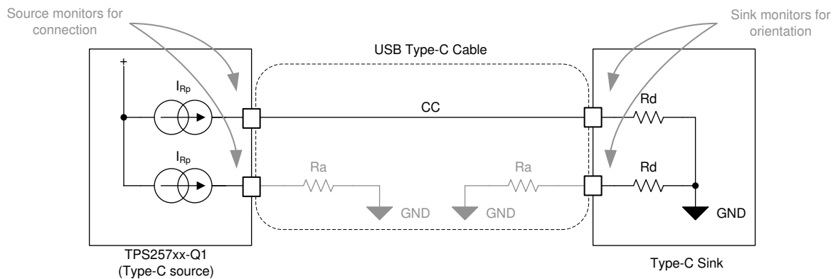
图 8-28. Type-C Cable
