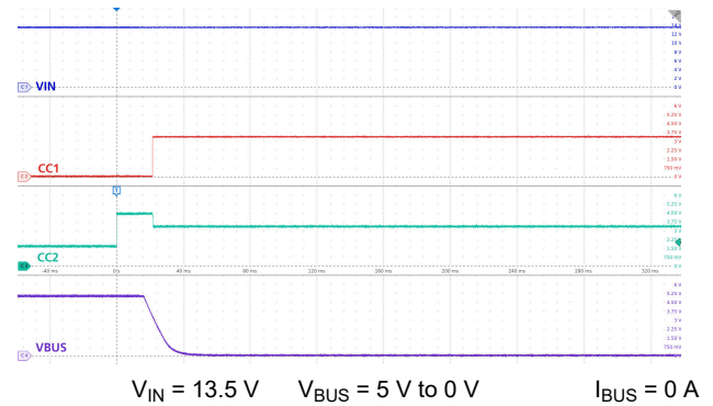
9-13. Type-C Detach
