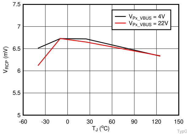
図 6-3. V RCP vs. Temperature
