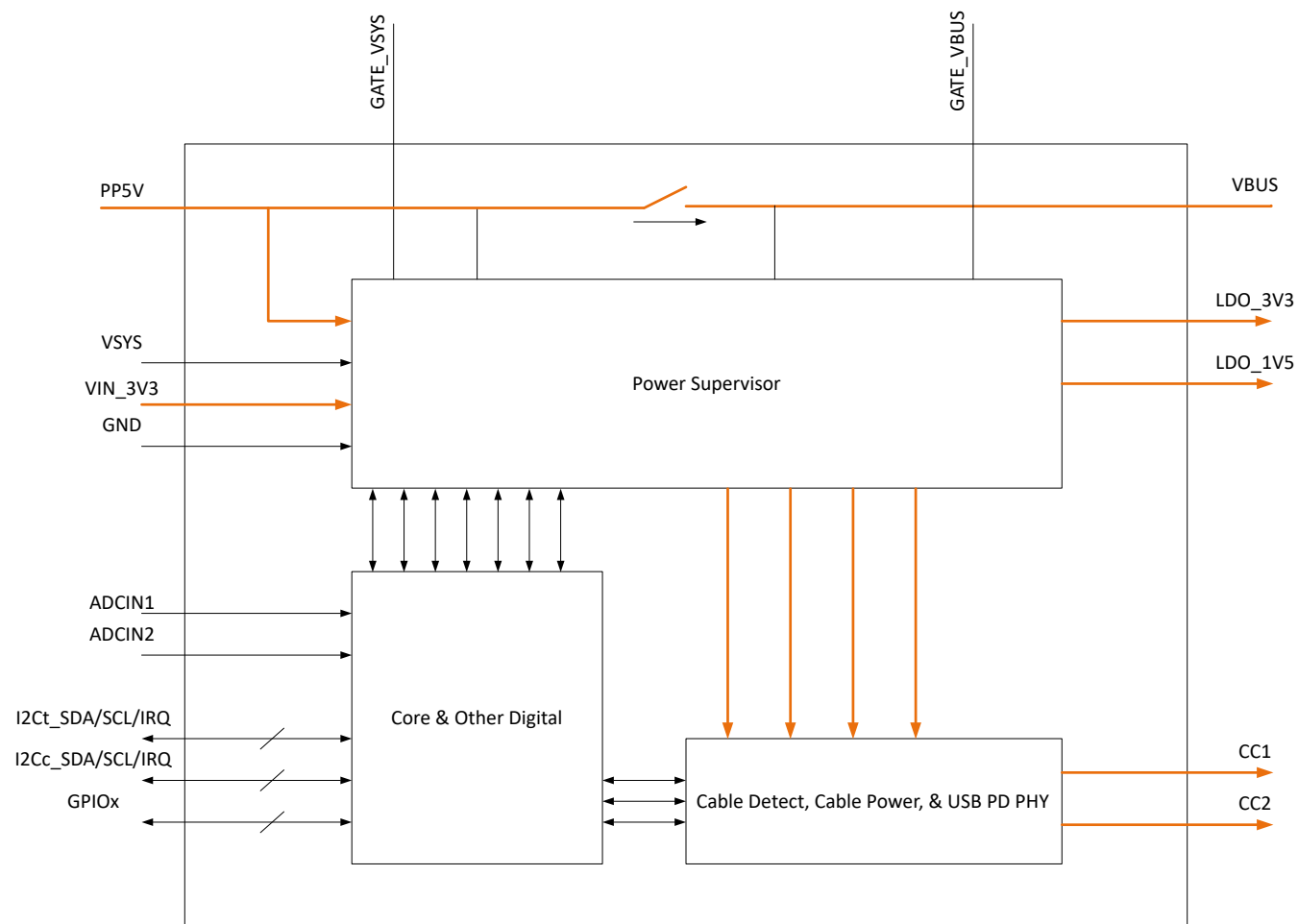
図 8-2. TPS25751S
