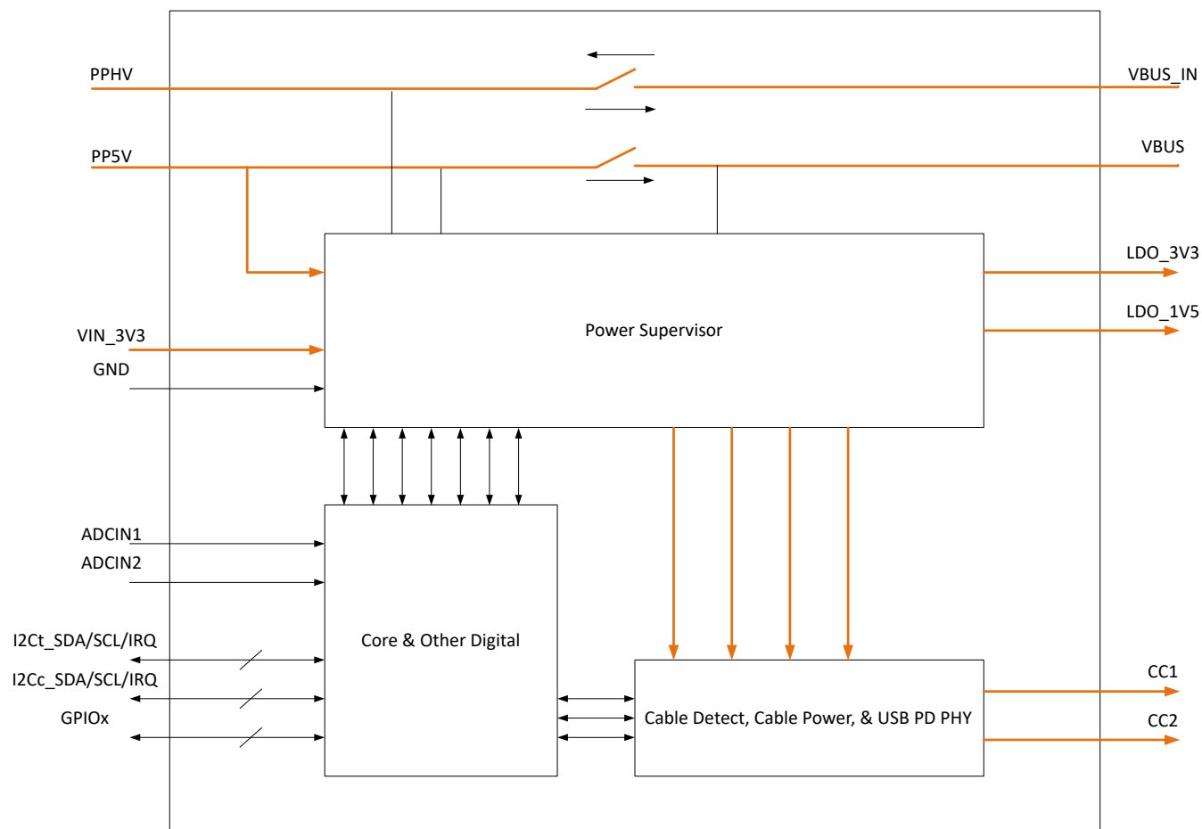
図 8-1. TPS25751D
