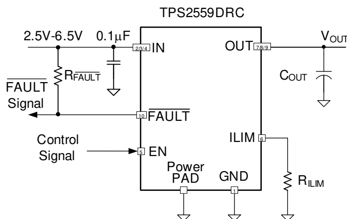
概略回路図
