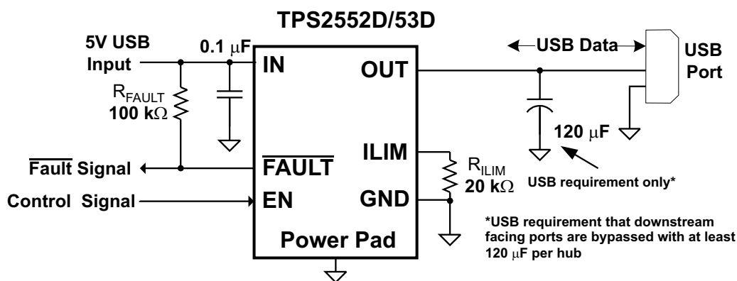
概略回路図
