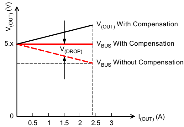
図 8-1. Voltage Drop
