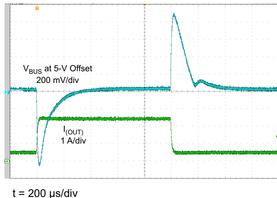
9-8. 0.5-A \leftrightarrow 2.4-A Load Transient With 100-mA/ \mu\text{s} Slew Rate, V_{BUS}
