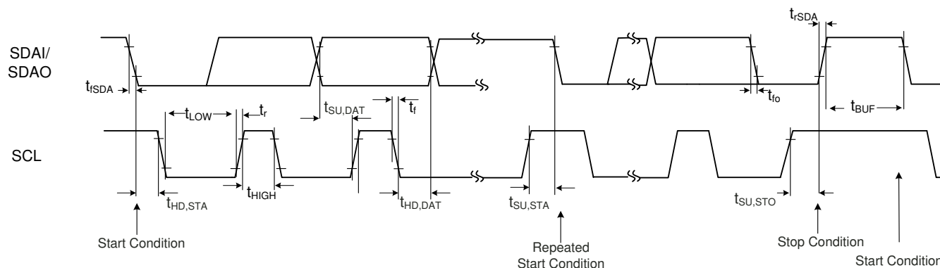
图 8-1. I²C Timings
